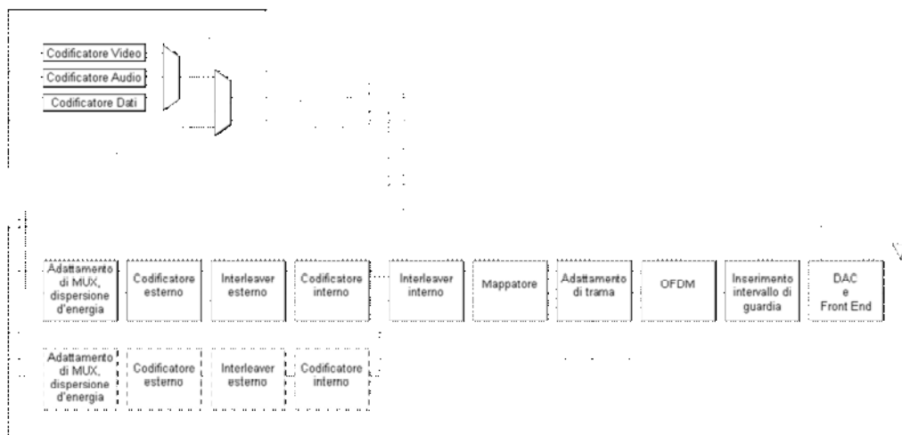
Figura 2 – Funzionamento di una rete DVB-T
