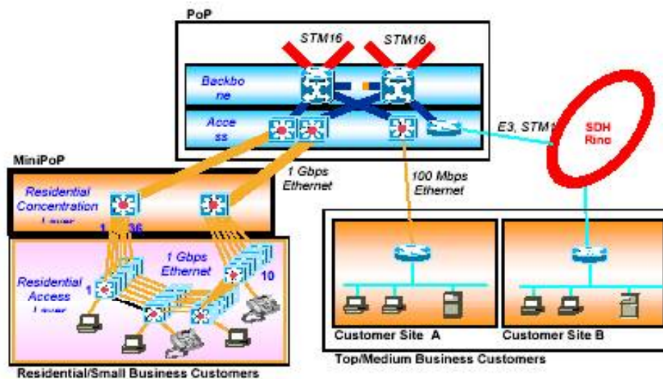
Figura 6 - Architettura Rete di Accesso
