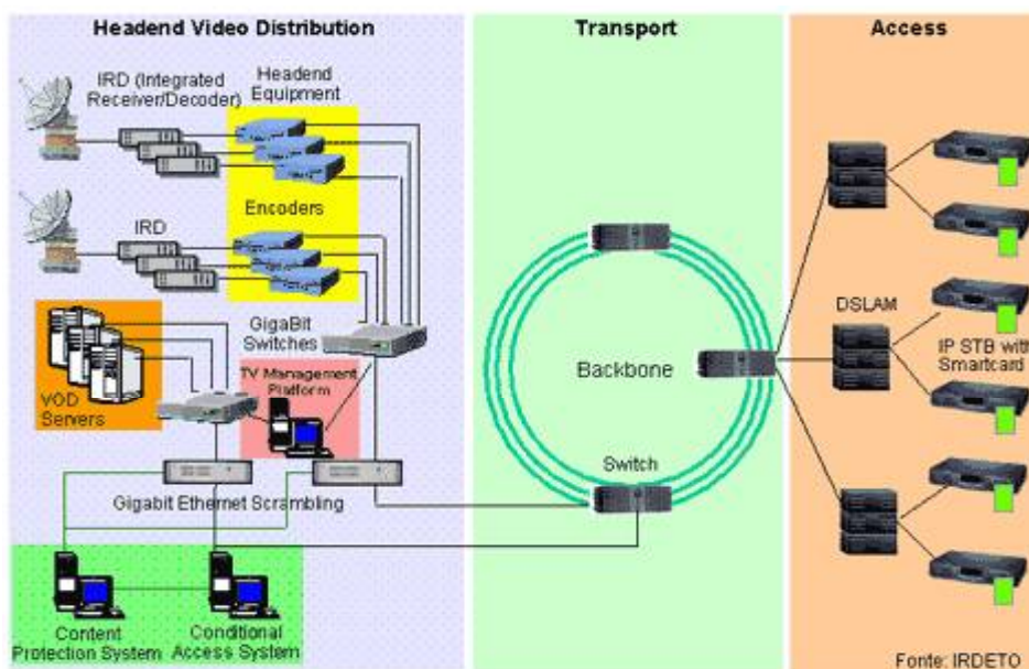
Figura 3 - Architettura semplificata IPTV
